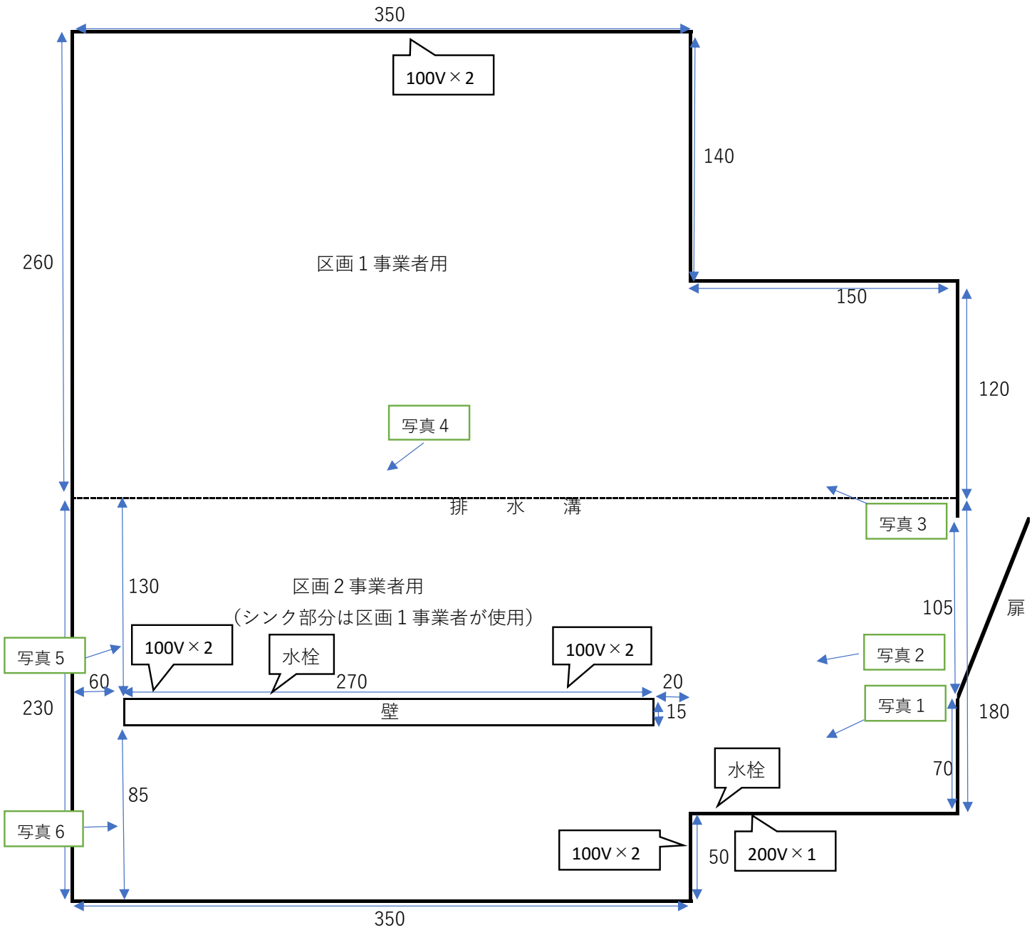
作業場レイアウト (概寸、cm)
